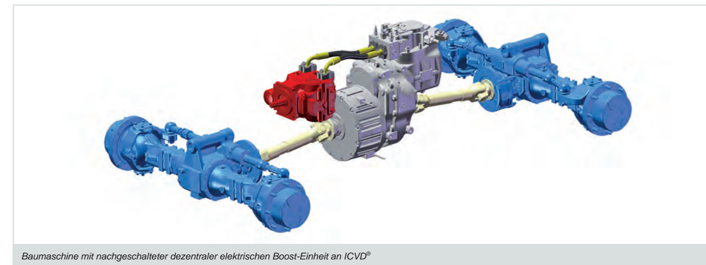
Baumaschine mit nachgeschalteter dezentraler elektrischer Boost-Einheit an ICVD®
