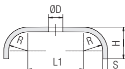
Tamaño STAUFF 1D hasta 3D
