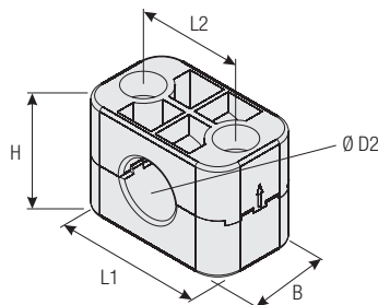
Para emplear con tubos flexibles compactos (Mitad de abrazadera superior girada 180°)
