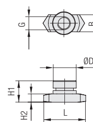
Tamaño STAUFF 2D hasta 5D
