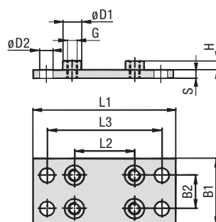
Tamaño STAUFF 10S hasta 12S
