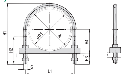
Abrazadera de estribo redondo (tipo RB) con zapata plástica (tipo RUL)
