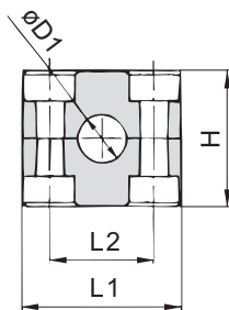
Tamaño STAUFF 1A hasta 8
