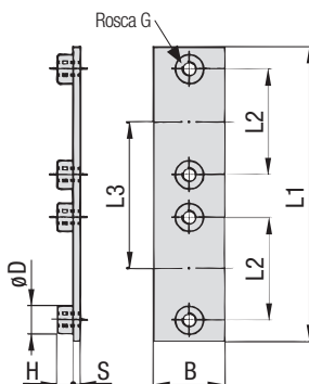
Tamaño STAUFF 1A hasta 8
