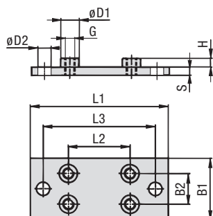
Tamaño STAUFF 3S hasta 9S
