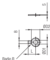
Chapa de seguridad SI
