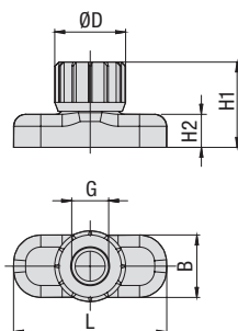
Tamaño STAUFF 1D
